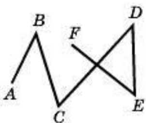
Ламана ABCDEF
