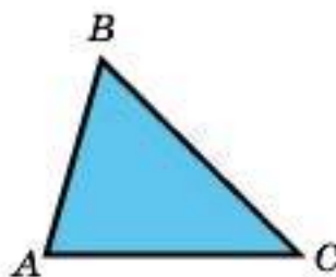
Трикутник ABC
